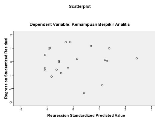
Gambar 1. Uji Heteroskedastisitas
