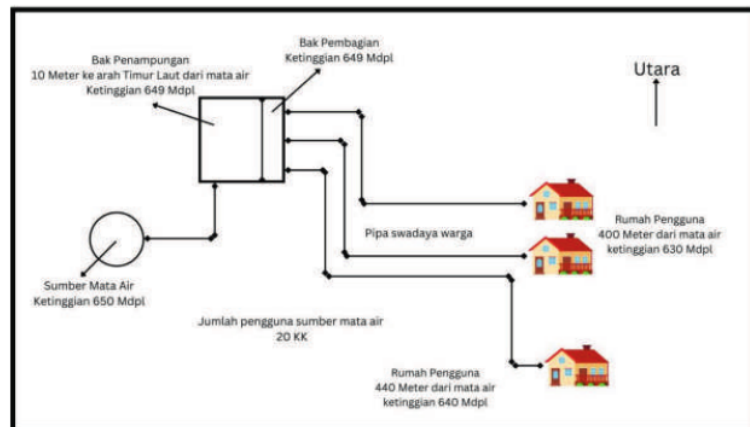
Gambar 10. Detail Engineering Desain Desa Pengung titik 2
