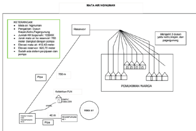
Gambar 9. Detail Engineering Desain Desa Petungsinarang Titik 2
