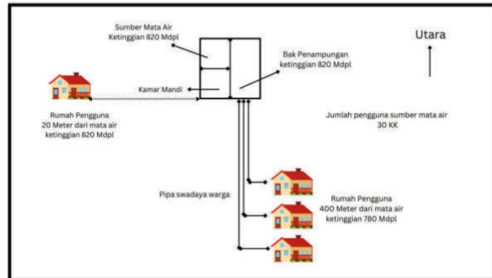
Gambar 9. Detail Engineering Desain Desa Pengung titik 1
