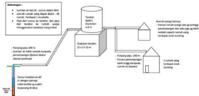
Gambar 3. Detail Engineering Desain Desa Sempu
