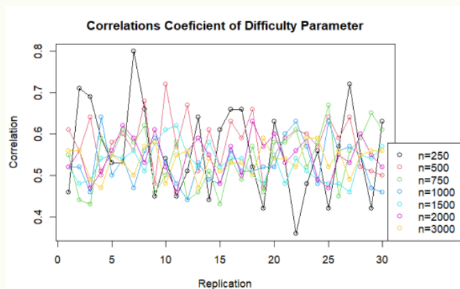
Gambar 4B. Korelasi dari Parameter Kesulitan
