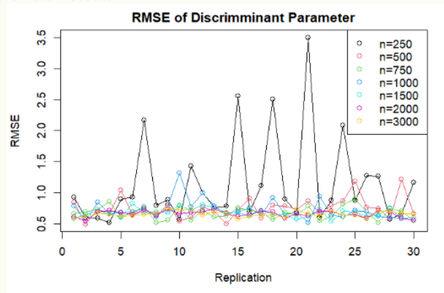
Gambar 3A. RMSE dari Parameter diskriminan
