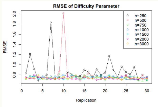
Gambar 3B. RMSE dari Parameter Kesulitan
