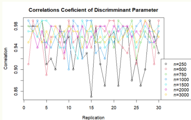
Gambar 4A. Korelasi dari Parameter diskriminan
