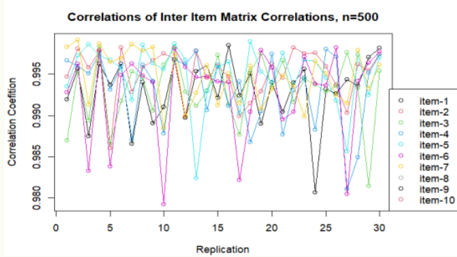
Gambar 2B. Korelasi antara matriks korelasi inter item dari data awal dengan data bangkitan n=500
