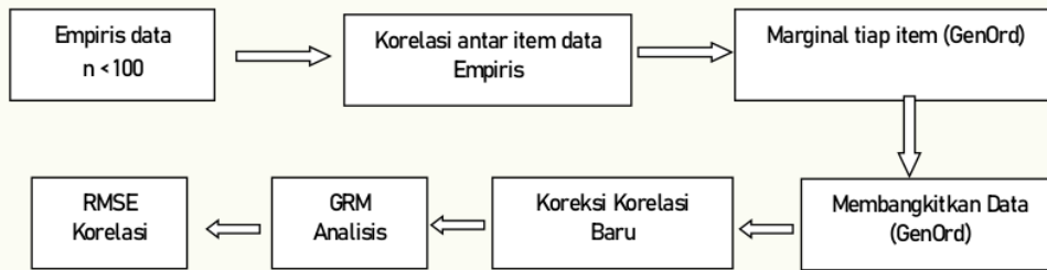
Gambar 1. Procedure estimasi parameter butir dan item fit
